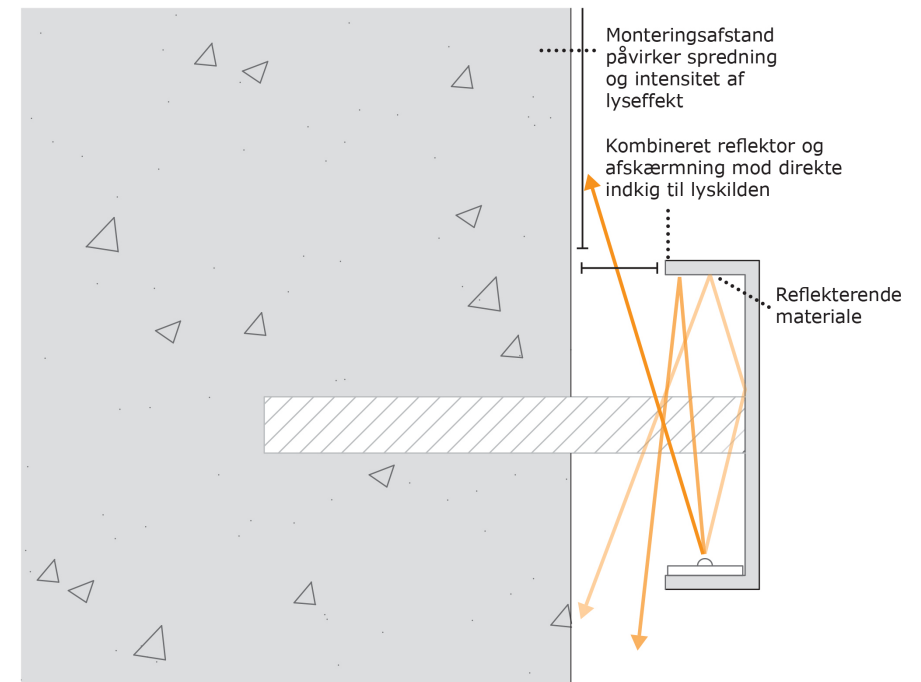
Fig. 8: Principsnit, der illustrerer, hvordan lyset distribueres.
