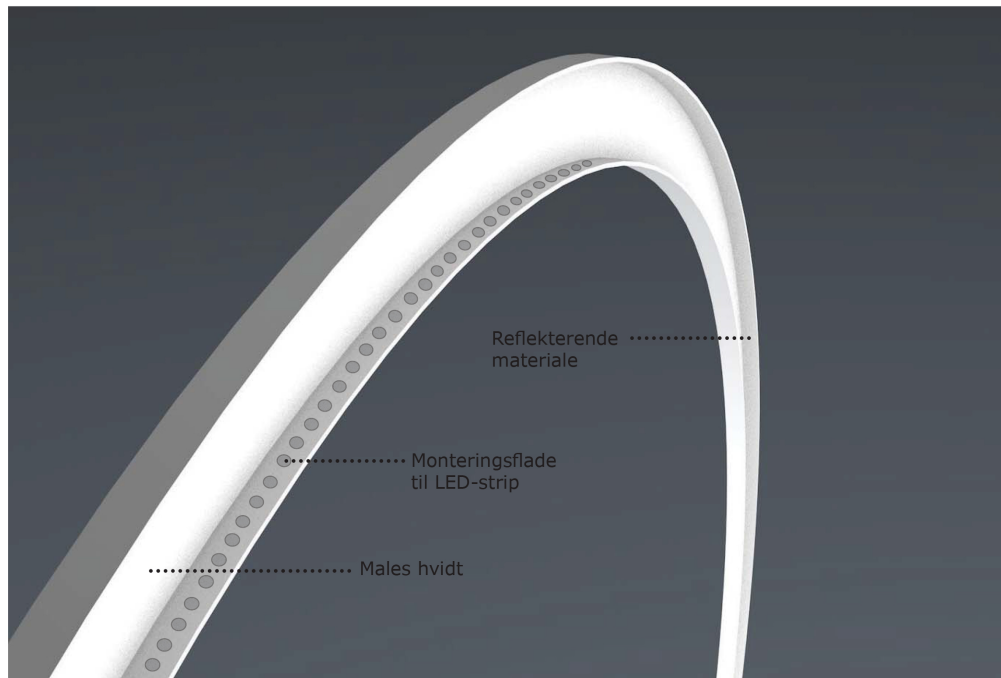
Fig. 7: Diagram: Konstruktionsprincip ved brug af valset U-profil i aluminium og LED-strip.
